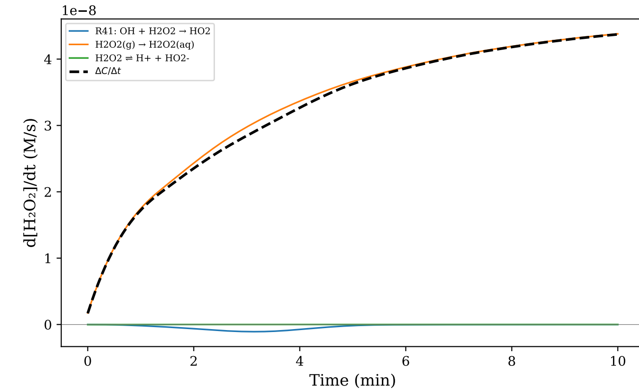
(d) \text{H}_2\text{O}_2
